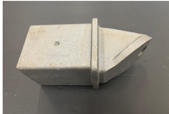
Hjørnestuss for 4-kt. åk med 4-kt. rør 100x4 og 104x6mm
