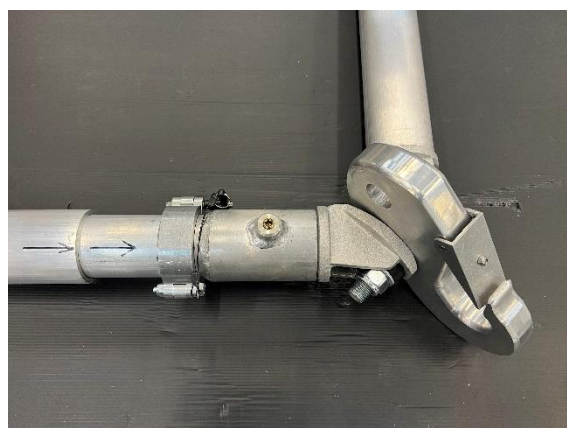
Firkant åk med stillbar løsning (runde rør). Det er dreide spor i røret for hver 25 cm. som klemmen kan flyttes til.
