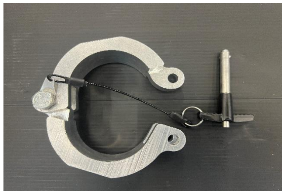
Lås for teleskop med rundt rør
